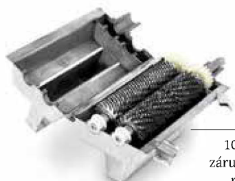
Nože manuálního tenderizéru.
